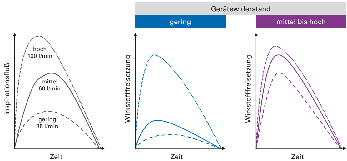
Abb. 2: Zusammenhang zwischen Flussrate, Gerätwiderstand und Wirkstofffreisetzung (modifiziert nach [19, 20])
