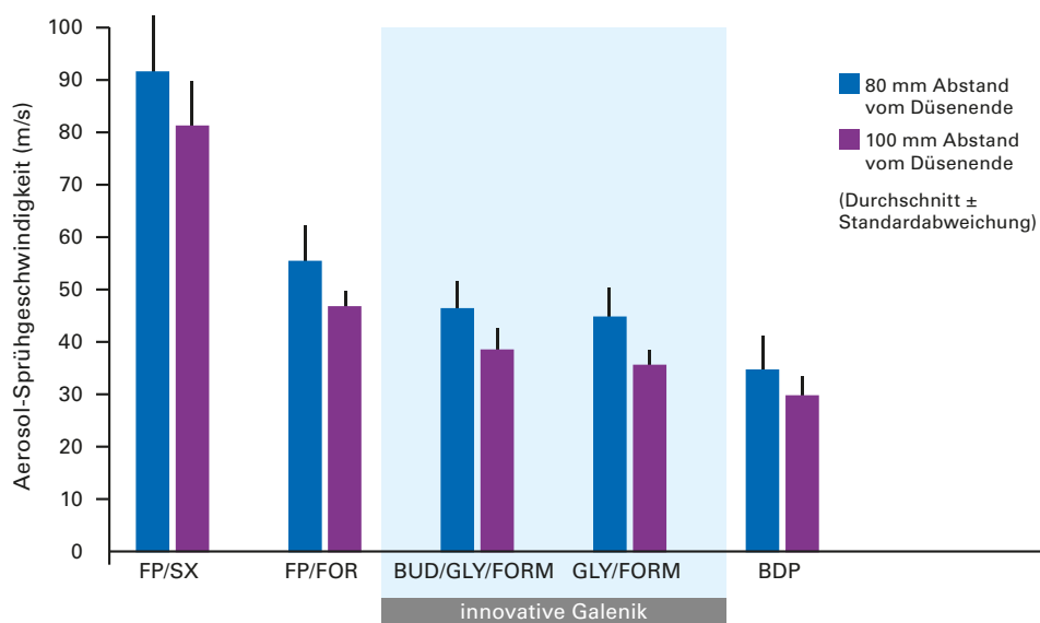
Abb. 5: Sprühgeschwindigkeiten (Mittelwert \pm SD) von zwei pMDI (BUD/GLY/FORM und GLY/FORM) unter Verwendung der innovativen Galenik mit aerodynamischen Trägerpartikeln und von drei weiteren pMDI mit FP/SX, FP/ FOR und BDP (modifiziert nach [32])
