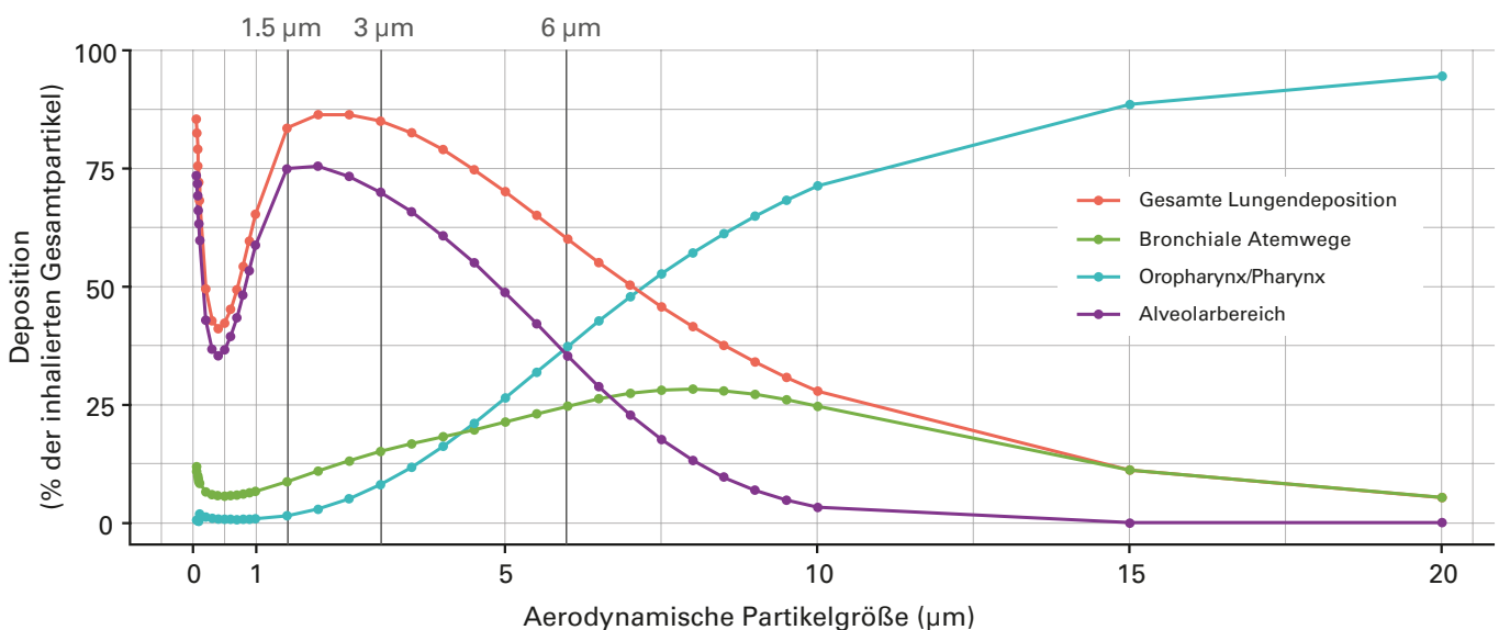
Abb. 3: Abhängigkeit der Lungendeposition von der Partikelgröße (modifiziert nach [15])
