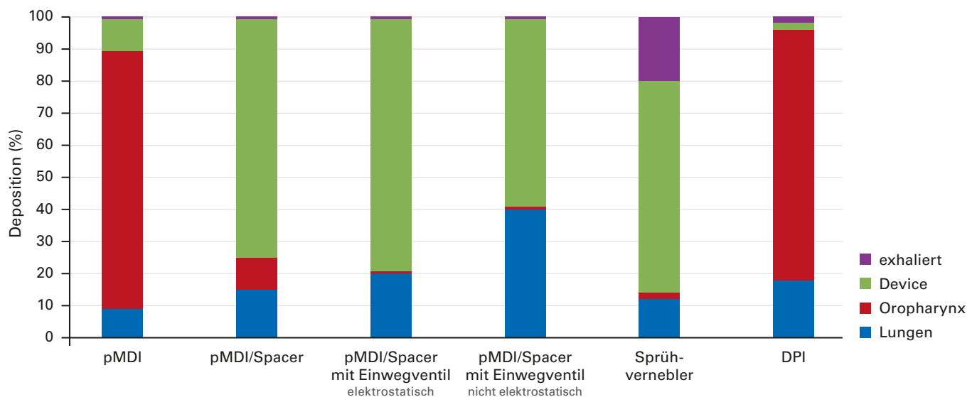
Abb. 4: Wirkstoffdeposition der verschiedenen Inhalationsgeräte: Farblich dargestellt sind die unterschiedlichen Prozentsätze der Lungendeposition und der Verluste im Oropharynx, im Device sowie beim Ausatmen (modifiziert nach [21])
